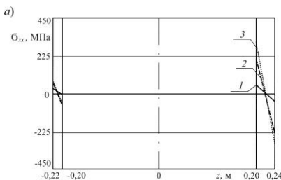
1 – фторопласт, 2 – пенопласт, 3 – пенополиуретан Рисунок 4. – Распределение нормальных напряжений по толщине пластины при изменении материала заполнителя в несущих слоях (а) и в заполнителе (б)
