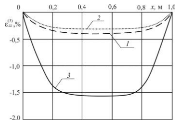
1 – упругая пластина, 2 – термоупругая, 3 – термоупругопластическая
